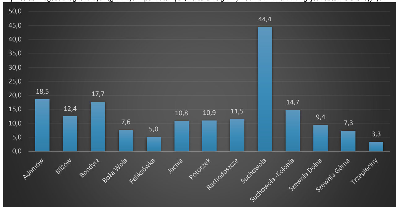
Wykres 65 Długość dróg lokalnych (gminnych i powiatowych) na terenie gminy Adamów w 2021 r. wg. jednostek referencyjnych
